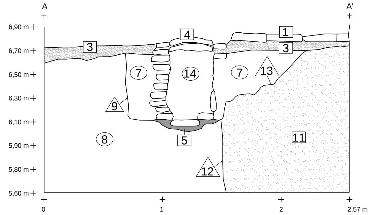
SECCIÓ A-A'
